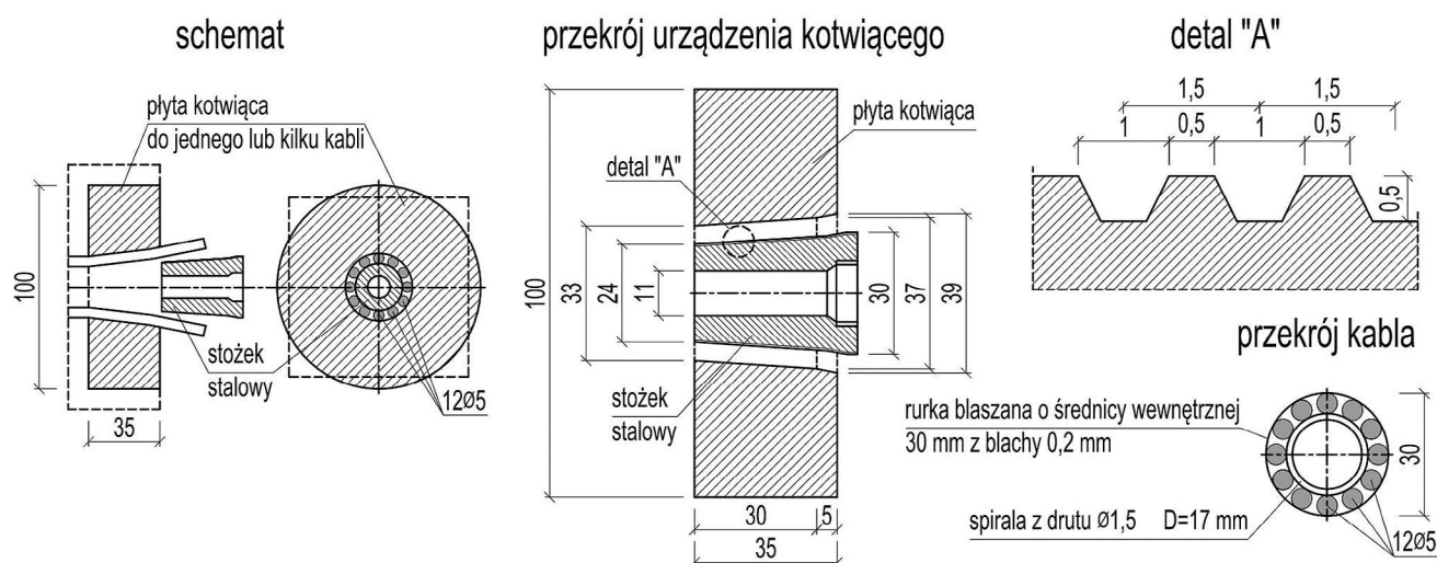
Rys. 4. Szczegóły stalowych bloków i stożków kotwiących według [10, 11]
