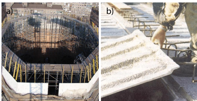
Rys. 8. Deskowanie tracone z GFRK: a) kopuła kościoła, Mariupol, Ukraina [38], b) stop [39]
