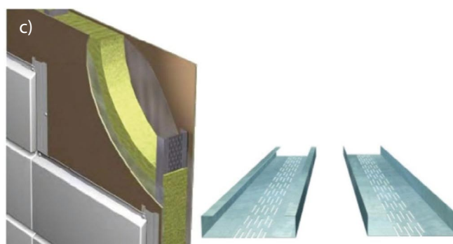
Rys. 4. Innowacyjne rozwiązania: a) wykorzystanie przestrzeni między żebrami płyty zespolonej do przepływu powietrza [M5], b) system fotowoltaiczny [M2], c) minimalizacja wpływu mostków cieplnych na słupkach ścian zewnętrznych [M5]
