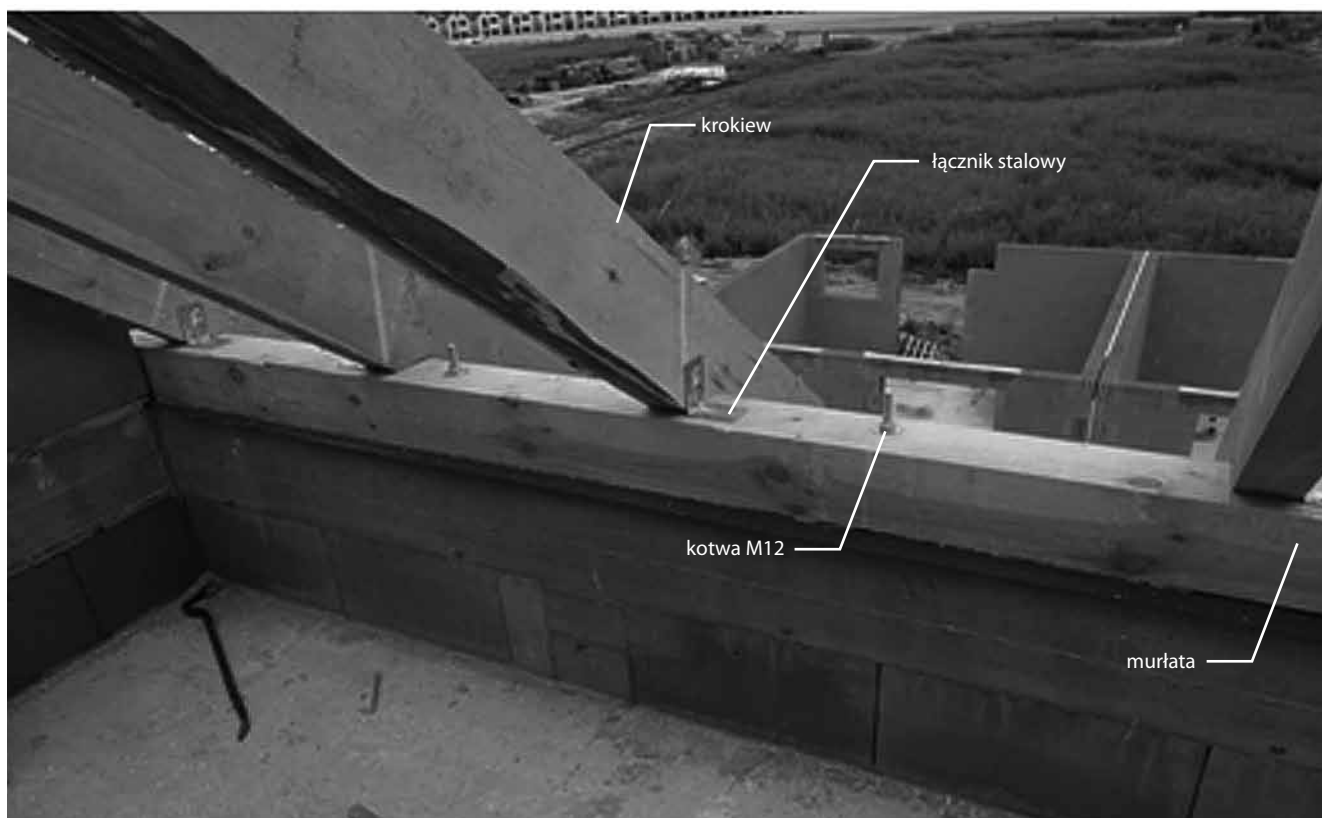
Rys. 4. Połączenie konstrukcji drewnianej dachu ze ścianami budynku
