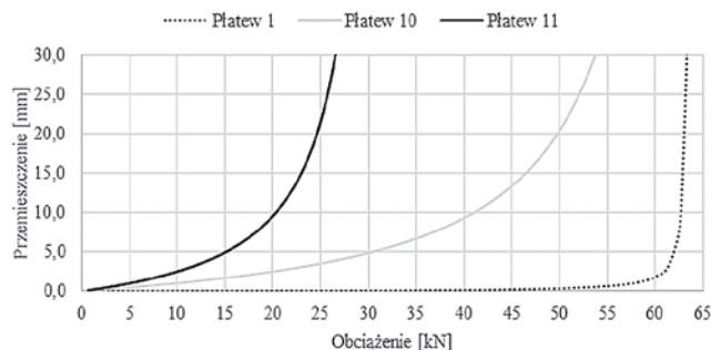
Rys. 3. Wykres przyrostu przemieszczeń do przyrostu siły – płatwę bazowa 1
