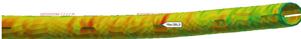
Rys. 7. Deformacja 6 płatwi z perforacjami
