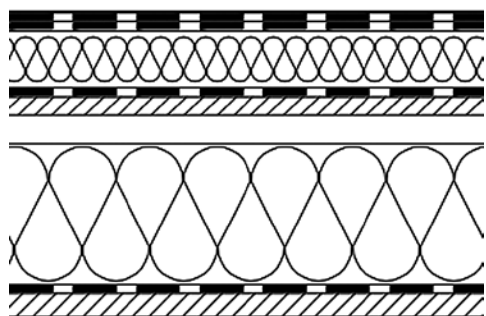
Rys. 1. Przekrój przez dach hali, warstwy od góry: papa nawierzchniowa termozgrzewalna, papa podkładowa, wełna mineralna twarda, paroizolacja, płyta OSB, pustka powietrzna wełna mineralna miękka, paroizolacja, deski strugane (archiwum autora)
