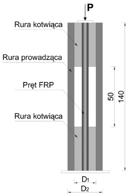
Rys. 3. Schemat badania pręta na ściskanie zgodnie z normą GOST [6]
