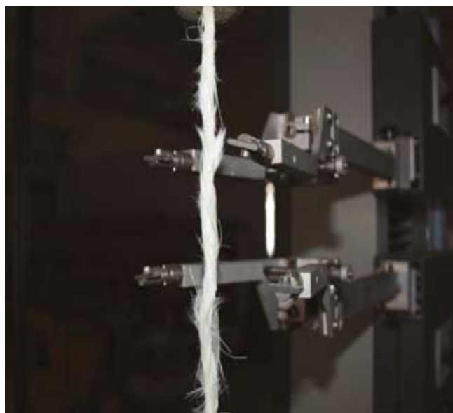
Rys. 2. Rozwarstwienie włókien na odcinku pomiarowym; widoczny ekstensometr pomiarowy o regulowanej bazie
