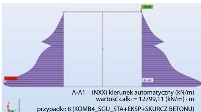
Rys. 4. Siły obwodowe od ciężaru własnego zbiornika, skurczu betonu i parcia wody
