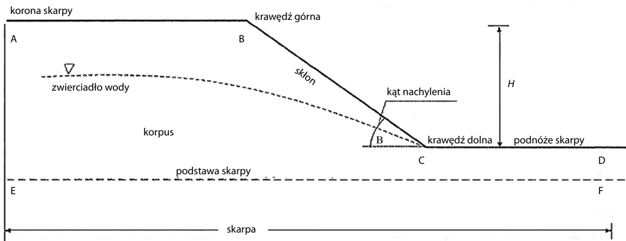
Rys. 2. Schemat sytuacyjny analizowanego zadania – skarpa A-D; korpus o objętości mas ziemnych ABCD i EFA; korona skarpy A-B o powierzchni płaskiej lub nieznacznie nachylona do skłonu; skłony B-C czyli linia spadku; podnóże C-D, czyli stopa, tj. część powierzchni skarpy poniżej skłonu; podstawa skarpy E-F, czyli granica zasięgu technicznie istotnych wpływów stanu naprężeń i odkształceń wywołanych istnieniem stoku i jego obciążenia; również zasięg osuwiska poniżej podnóża; kąt nachylenia stoku (b), czyli kąt nachylenia linii skłonu do poziomu oraz wysokość H jako długość rzutu odcinka BC na oś pionową
