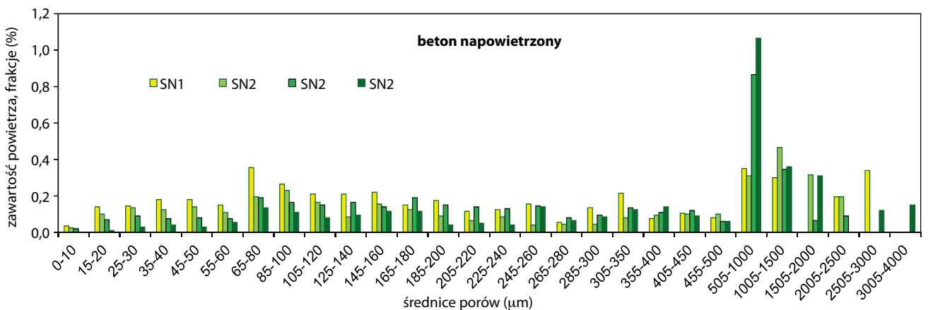
Rys. 6. Rozkład wielkości porów w betonach napowietrzonych
