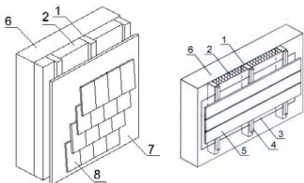
Rys. 3. Schemat montażu elewacji drewnianej: 1) łąty główne, 2) izolacja termiczna, 3) folia wiatrochronna, 4) łąty, 5) deski, 6) ściana nośna, 7) płyta OSB, 8) gont elewacyjny
