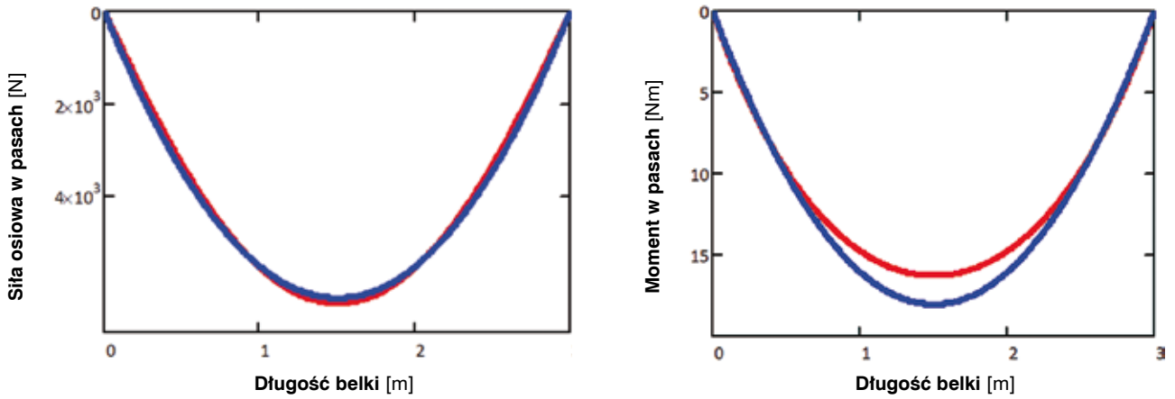
Rys. 18. Porównanie rozkładu siły osiowej i momentu zginającego w pasach drewnianych. Wykres czerwony przedstawia wartości policzone metodą Pischla, wykres niebieski wartości policzone metodą \gamma
