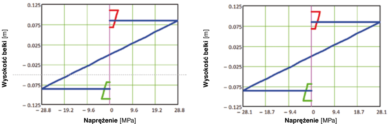
Rys. 20. Rozkład naprężeń w przekroju środkowym belki dla analizy metodą \gamma (lewa) i metodą Pischla (prawa)
