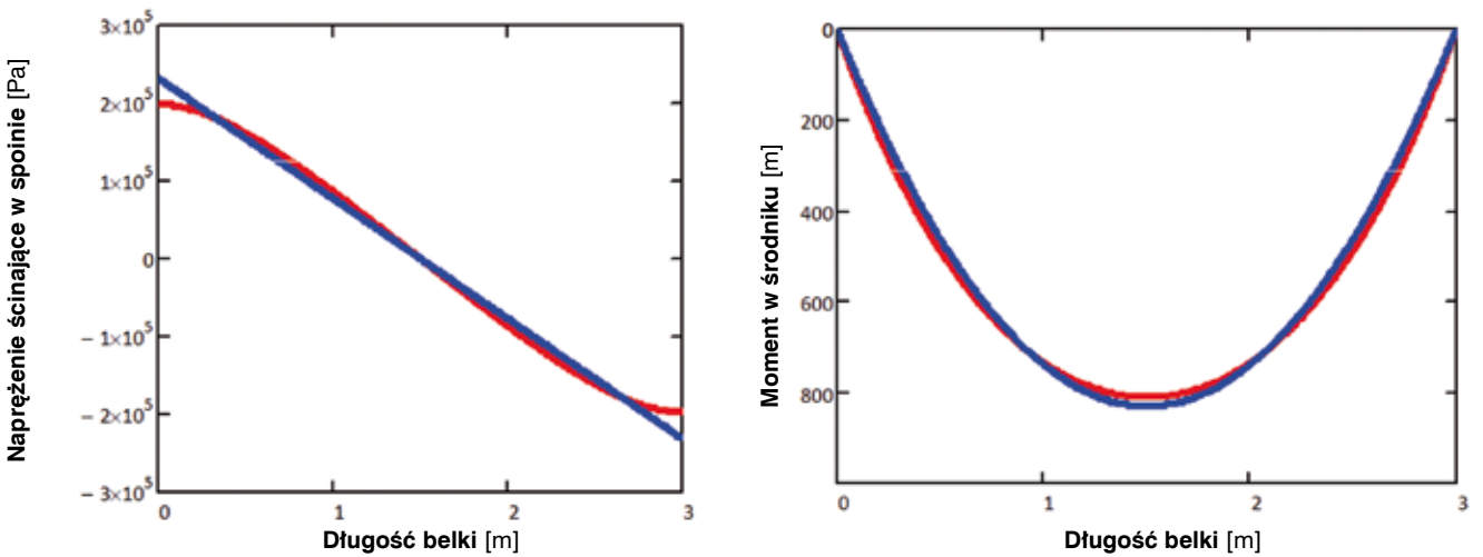
Rys. 19. Porównanie rozkładu naprężenia ścinającego w spoinie i momentu zginającego w środkniku szklanym. Wykres czerwony przedstawia wartości policzone metodą Pischla, wykres niebieski wartości policzone metodą \gamma
