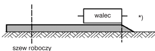
Rys. 7. Schemat wałowania nawierzchni pasami – formowanie szwu i krawędzi [1]
