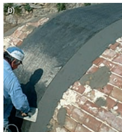
Rys. 1. Zbrojenie ściany murowanej (a) i sklepienia ceglano (b) materiałami FRCM [5]
