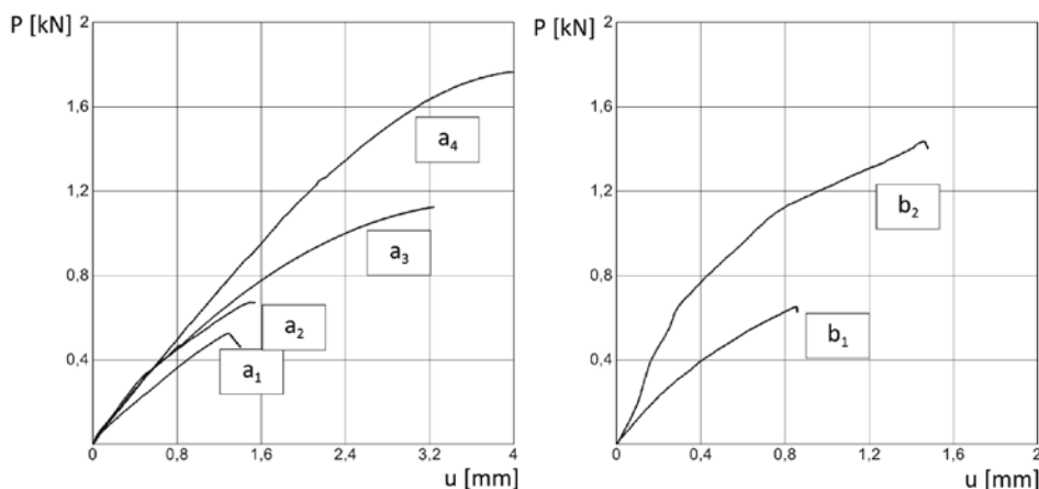
Rys. 4. Zależności między ugięciem „u” a obciążeniem „P” wybranych próbek zginanych z płaszczyzny ściany wzdłuż (a) i w poprzek (b) spoin wspornych
