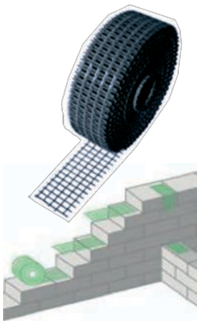
Rys. 2. Zbrojenie muru w cienkich spoinach siatkami kompozytowymi
