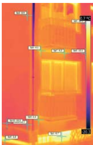
Rys. 14. Termogram do rysunku 13 (foto archiwum autora)
