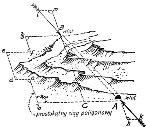
Rys. 4. Przypuszczalny sposób, w jaki Eupalinos wytyczył trasę tunelu pod maszyem góry Kastro na wyspie Samos w VI w p.n.e. (za [3])
