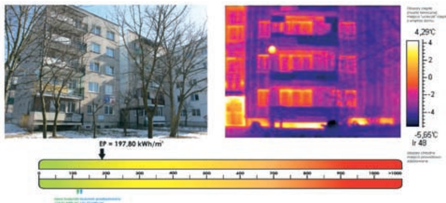
Rys. 4. Charakterystyka budynku reprezentatywnego (oprac. A. Ostańska 2010–11)
