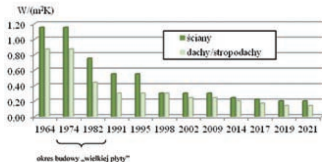
Rys. 2. Wymagane i planowane wartości współczynnika przenikania ciepła ścian i dachów/stropodachów w kolejnych wydaniach norm i przepisów krajowych
