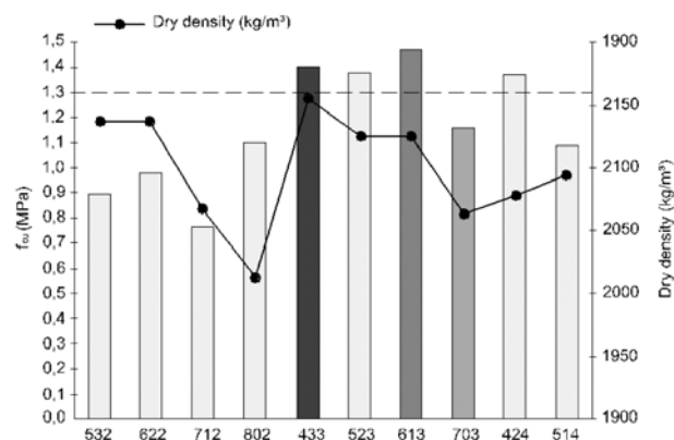
Rys. 3. Zależność między gęstością w stanie suchym a wytrzymałością na ściskanie dla różnych niestabilizowanych mieszanek ziemi [5]
