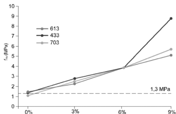
Rys. 4. Zależność między zawartością cementu a wytrzymałością na ściskanie dla próbek z trzech różnych rodzajów ziemi [9]
