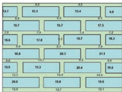
Rys. 7. Rozprzestrzenianie się wody w murze ceglany. Do budowy została użyta porowata zaprawa. Wielkości podane w diagramie oznaczają ilości wody mierzone procentowo w stosunku do masy cegły/zaprawy [15]
