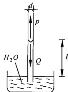
Rys. 4. Podciąganie kapilarne [12]
